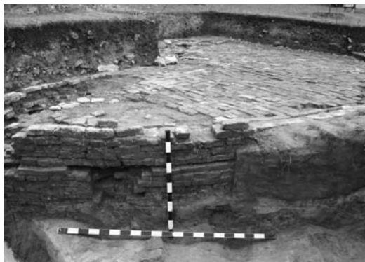
Илл. 4. Западный фонтан «против гrotцев». Глиняный замок в основании и с внешней стороны сооружения. Характер кладки. Вид с запада
